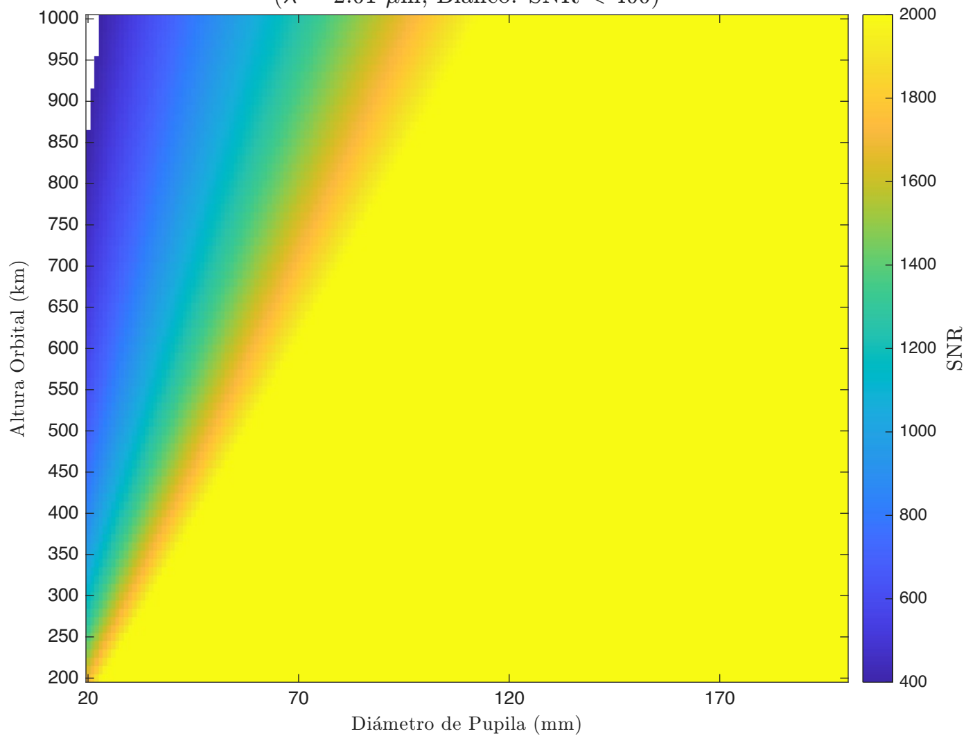
SNR - TMA - Detector 3 ( \lambda = 2.01 \mu\text{m} , Blanco: SNR < 400)
